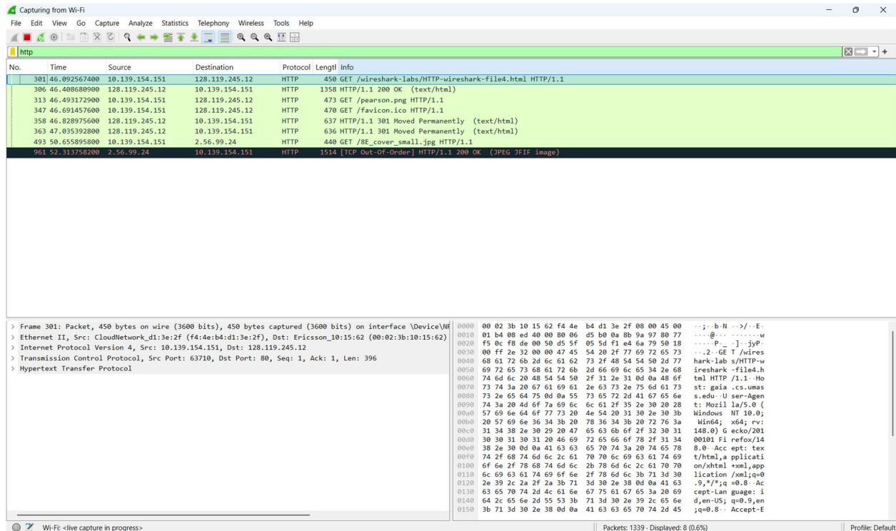
Gambar 4.4 hasil penangkapan paket HTTP menggunakan aplikasi Wireshark ketika browser mengakses halaman HTTP-wireshark-file4.html.
