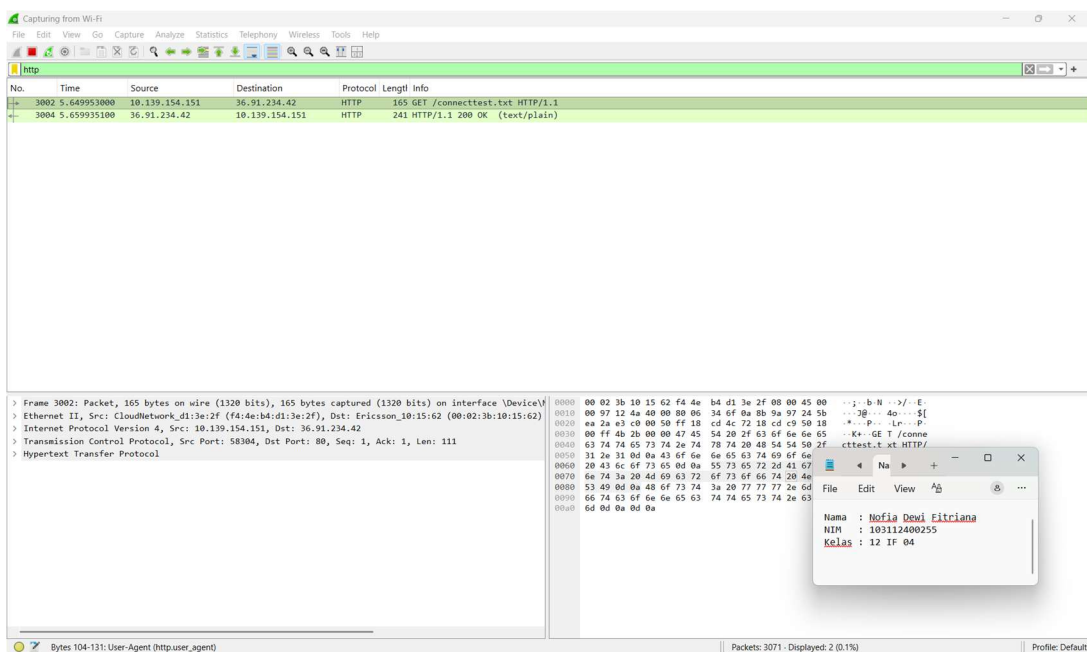
Gambar 2.2 tampilan Wireshark yang menunjukkan request dan response HTTP sederhana.
