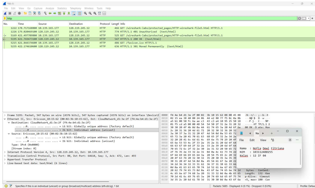
Gambar 5.5 menunjukkan hasil penangkapan paket HTTP menggunakan aplikasi Wireshark ketika mengakses halaman yang dilindungi autentikasi.
